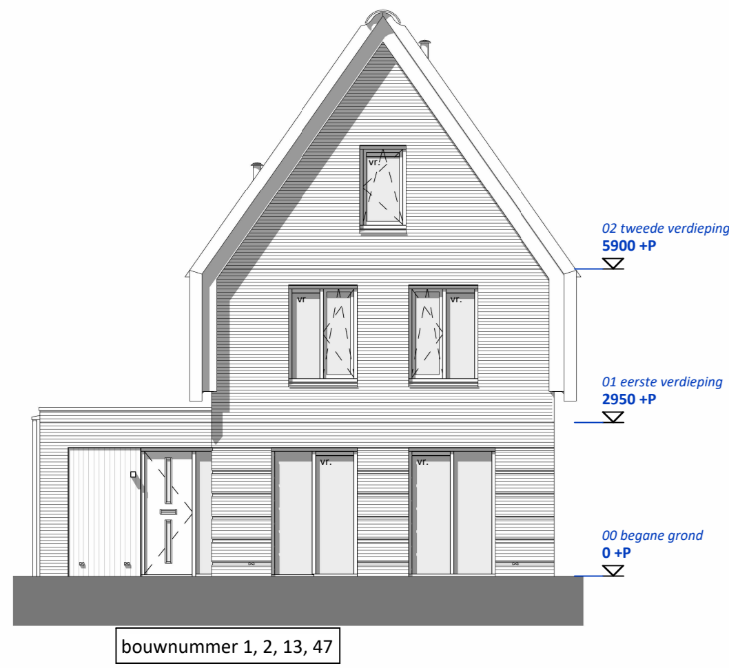
voorgevel V sp 1 : 100
